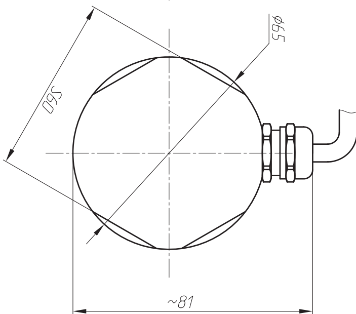
Габаритные размеры ТЛ-С1 тип 2 с присоединением "кабель" ТВп(L) (L) - длина кабеля в метрах
