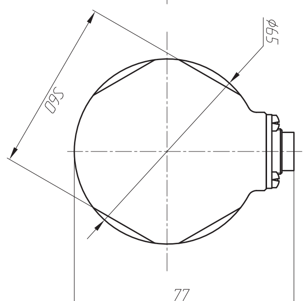
Габаритные размеры ТЛ-С1 тип 2 с присоединением "разъем" С60(L); С70(L); С80(L) (L) - длина кабеля в метрах
