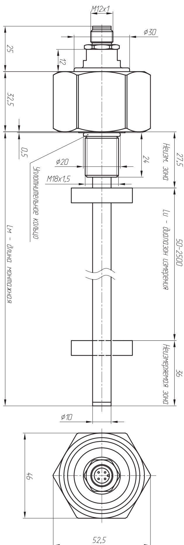
Габаритные размеры ТЛ-СВ2 с присоединением «разъем» (С40(L))
