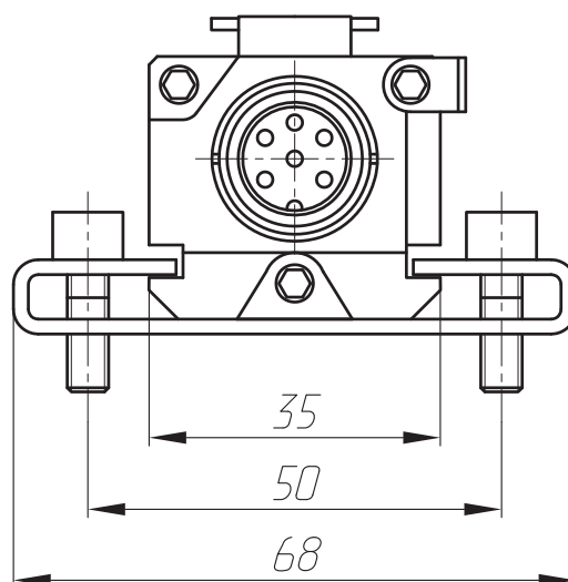
Габаритные размеры ТЛ-ПЗ с присоединением "разъем" С60(L); С80(L) (L) - длина кабеля в метрах
